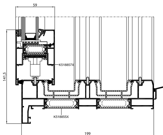
Przekrój drzwi z ościeżnicą 3-szynową
