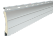
PA 45 wysokość profilu: 45 mm grubość: 9 mm
